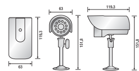
Night Vision Camera(Metal) : SOC-N121
